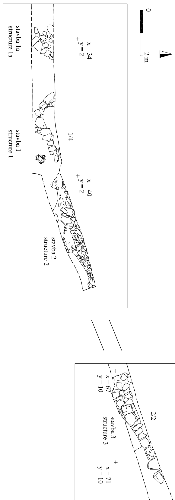
Sl. 4: Most na Soči – Maregova gura. Tloris sond 1/4 in 2/2 z vrisanimi stavbnimi ruševinami. M. = 1:100.
