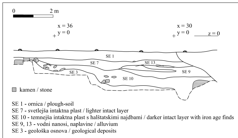
Sl. 5: Most na Soči – Maregova gura. Južni profil v sondi 1/4. M. = 1:100.
