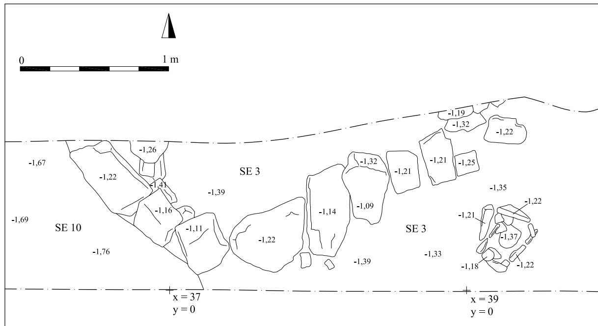
Sl. 6: Most na Soči – Maregova gura, sonda 1/4. Tloris stavbne ruševine 1 z jamo za stojko. M. = 1:25.
