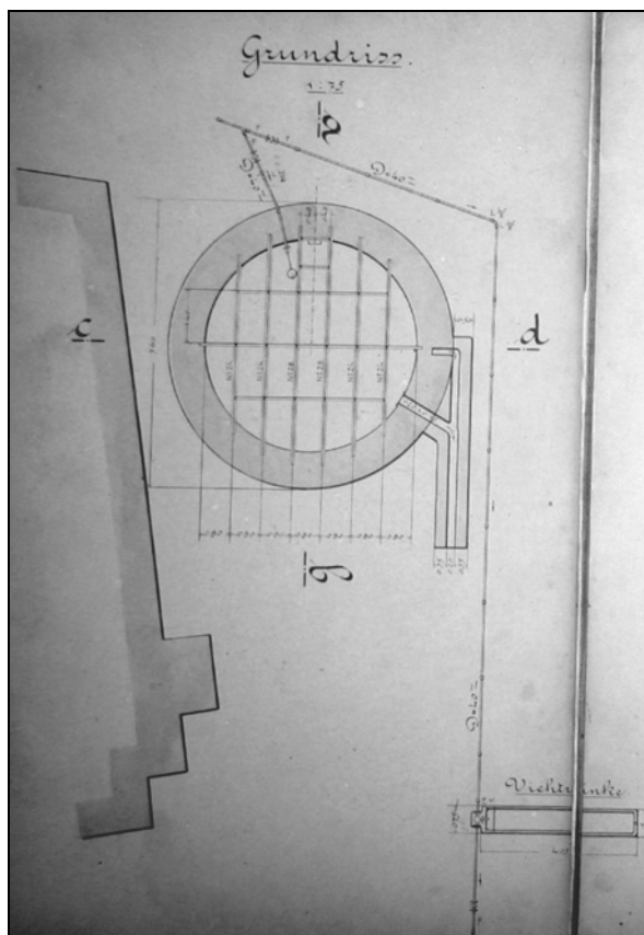
Tloris vodnega zbiralnika v vasi pred zgraditvijo vodovoda. Levo je zarisana zadnja fasada sosednje domačije Anžinovič, Dane 17 (SI PAK, KP 633, š. 472).
