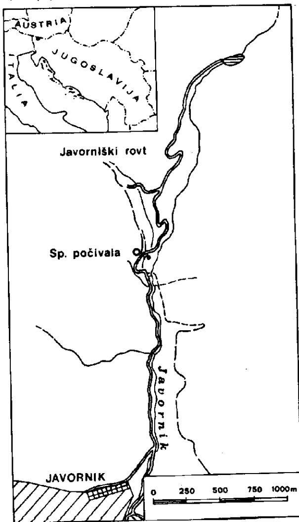
Фиг. 1. Скица местонахождения верхнекаменноугольных двустворки у Яворницком роуту
