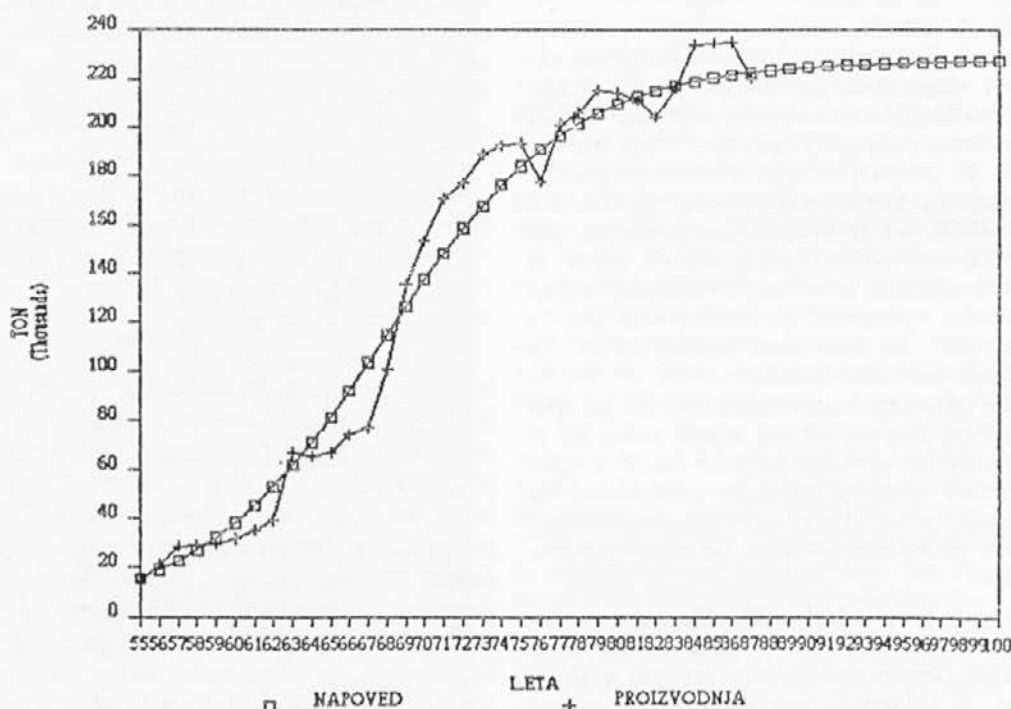
Slika 2: Razvoj proizvodnje v Jeklarni od leta 1955 dalje
