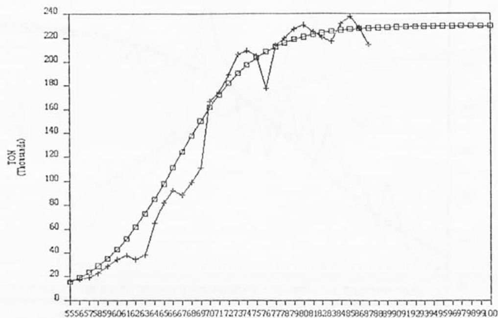
Slika 4: Razvoj proizvodnje v Valjarni od leta 1955 dalje
