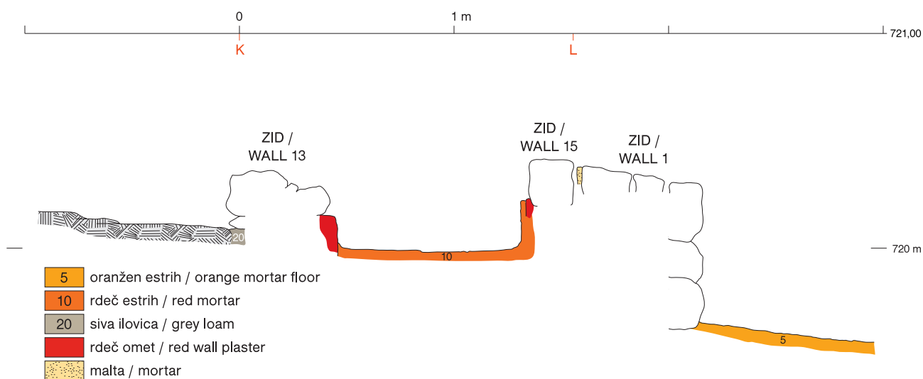
Sl. 2.46: Cerkev. Krstilnica, presek 6 (K-L; prim. sl. 2.29). M. = 1:25.
