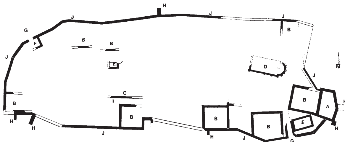
Sl. 12.26: Korintija. Tloris poznoantične utrdb (Tomičič 1986–1987, sl. 9).
