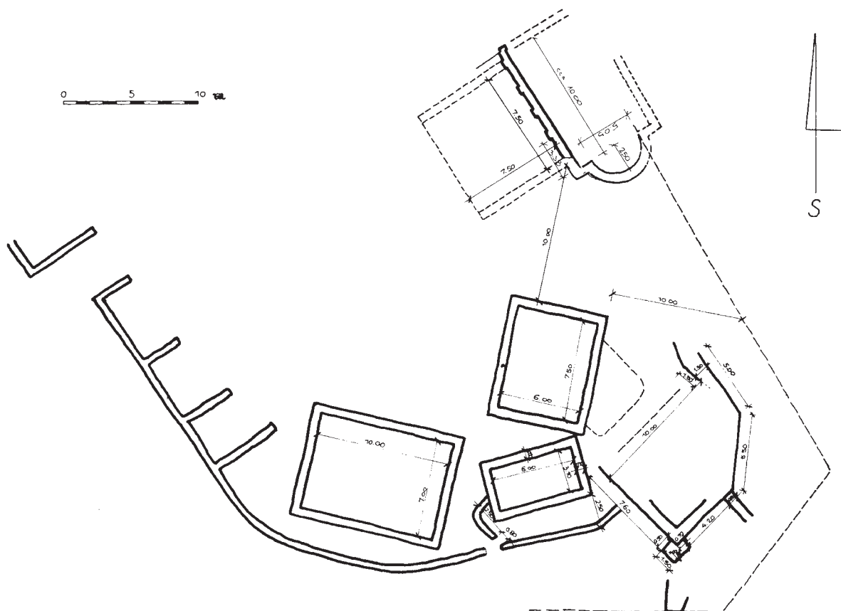
Sl. 12.25: Korintija. Tloris jugovzhodnega dela utrdb (Faber 1986–1987, sl. 13).
