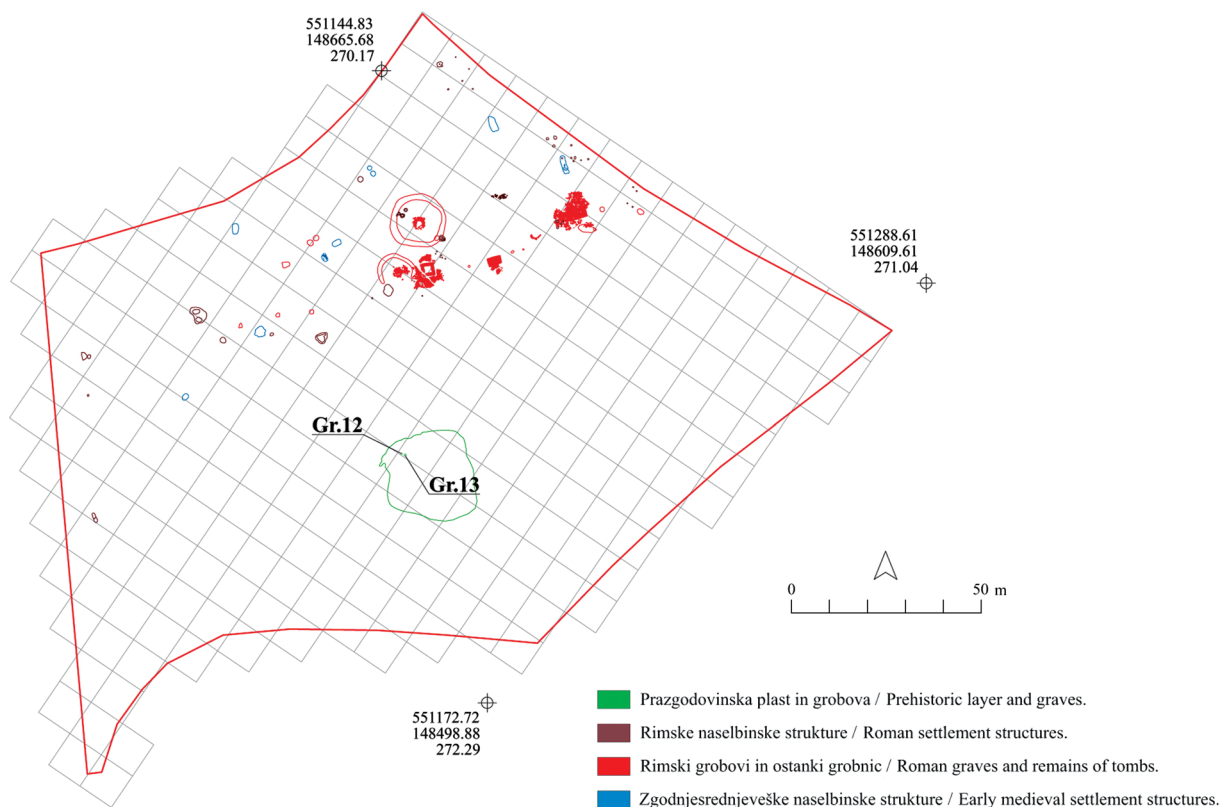
Sl. 3: Slivnica 3B – načrt najdišča z označenimi prazgodovinskimi, rimskodobnimi in zgodnj srednjeveškimi ostanki. Fig. 3: Slivnica 3B – site plan with marked Prehistoric, Roman and Early Medieval remains. (koordinatni sistem / coordinate system: D48/GK)
