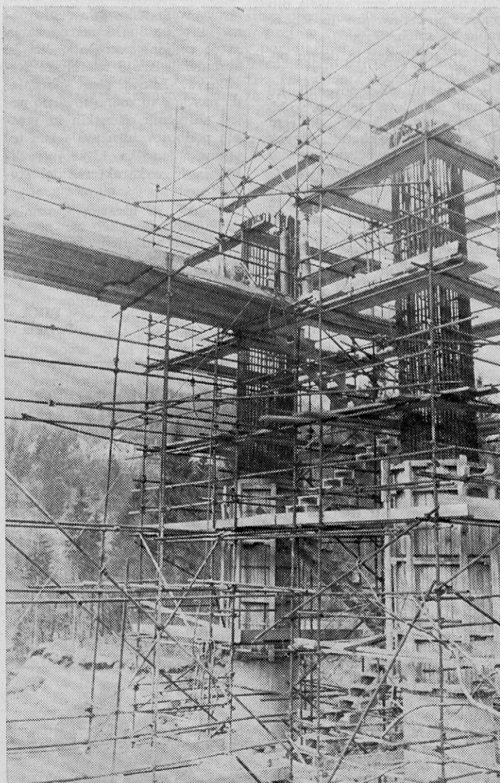
Železobetonska stebra bodočega mostu nove bohinjske ceste na Obrniah Na treh parih takih mostov bodo ležali jekleni nosilci in betonska plošča enega od obeh mostov zadnjega odsega ceste foto Ažman
