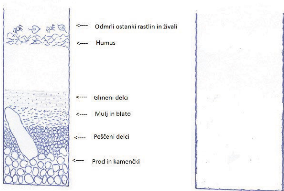
Slika 25: Porazdelitev delcev v prsti v vodnem stolpcu
