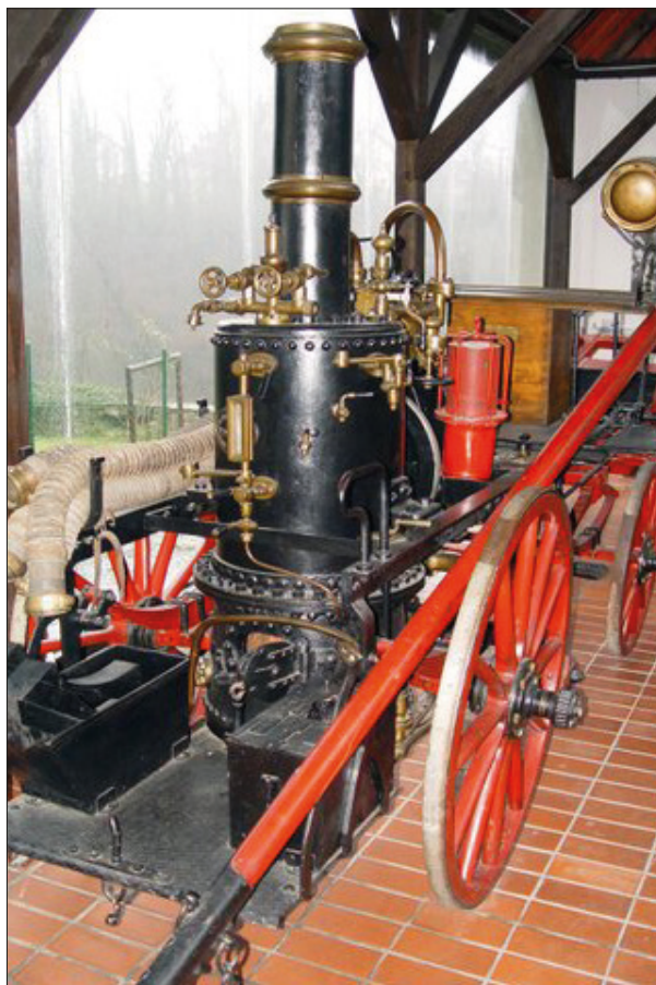
Parna brizgalna na vozu na konjsko vprego, 1908, eksponat v Slovenskem gasilskem muzeju dr. Branka Božiča Metlika
