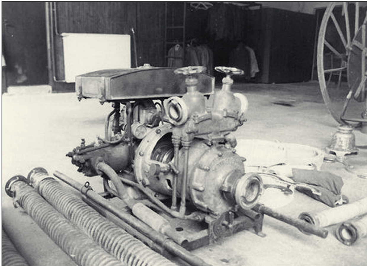
Eksponat iz Muzeja gasilstva Dravinjske doline: brizgalna Rosenbauer na motorni pogon, 1920
