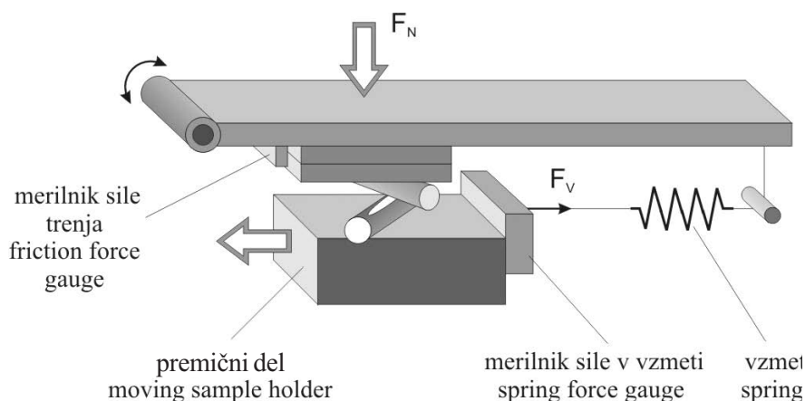
Sl. 1. Shematični prikaz naprave za tribološko preizkušanje
