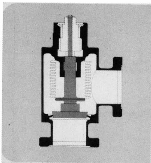
Slika 1.: Zaprt ventil
