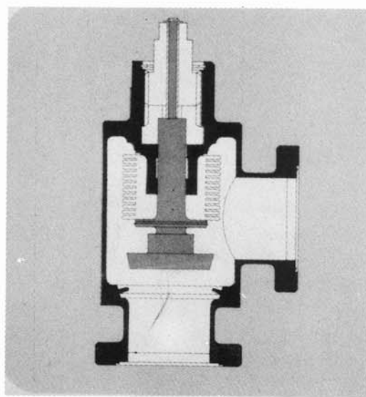
Slika 2.: Odprt ventil
