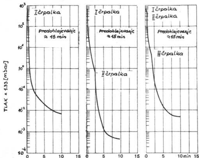
Sl. 3. Ena sorpcijska črpalka črpa volumen 46 litrov Dve sorpcijski črpalke črpata volumen 100 lit. Tri sorpcijske črpalke črpajo volumen 180 lit.
