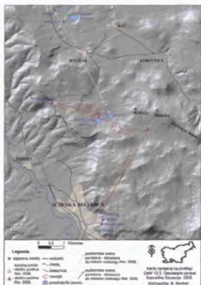
Podzemne vodne povezave, dokazane v zaledju Bistrice, Podstenjška in Pivke
