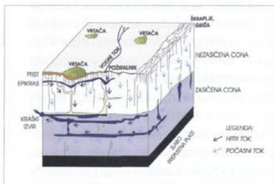
Shematski prikaz pretakanja vode v krasu (prirejeno po Doerfliger, Zwahlen, 1998)
