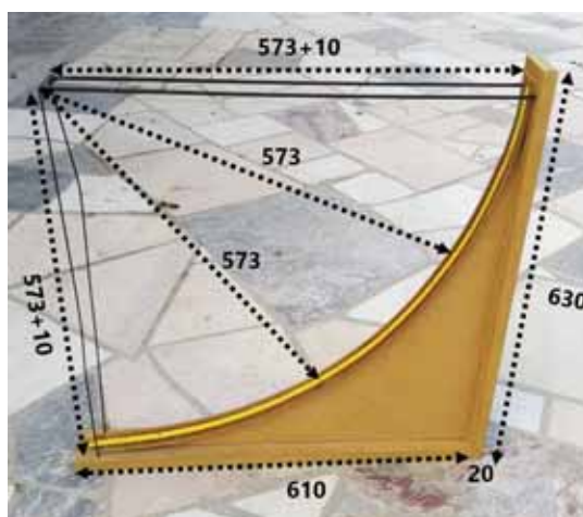
Slika 6: Kako izdelati sončni višinomer? Mere so v milimetrih. Prečka (polmer kroga) mora biti dolga 57,3 centimetra, saj bo tako ena stopinja ustrezala 1 centimetru na lestvici.
