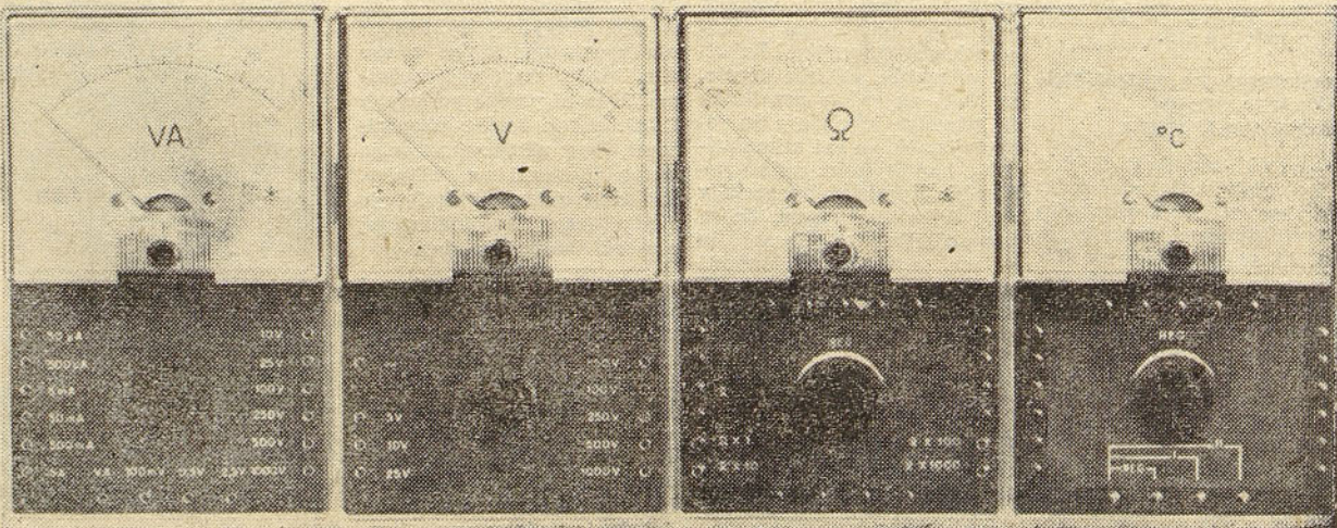
Izdelek Iskrine tovarne v Otočah (od leve): temperaturni merilnik s termistorjem tip TS 6A; ohmometer tip OS 6A; voltmeter za izmenični tok tip CS 6A; voltampermeter za enosmerni tok tip BS 6A
