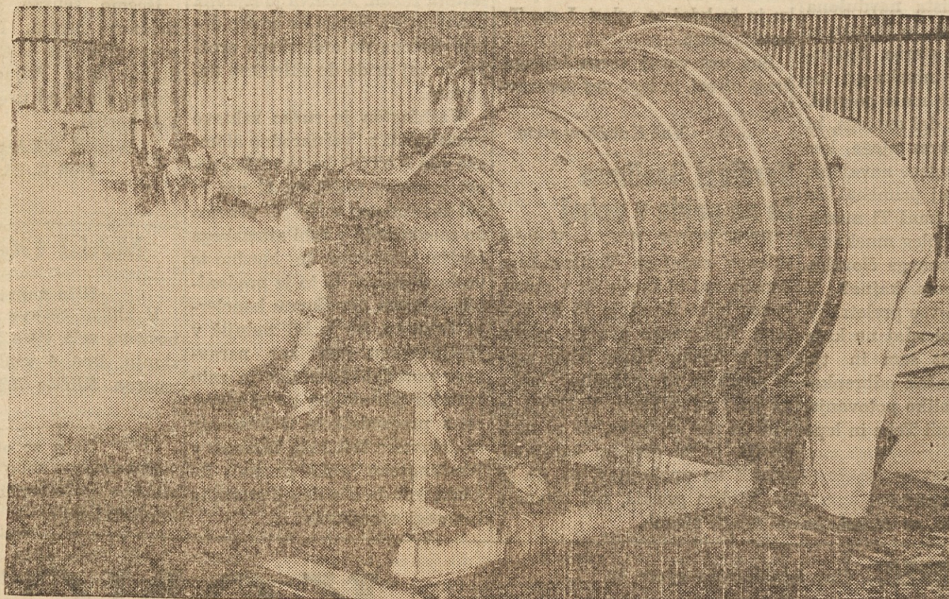
RAKETNI MOTOR TITANA — Tehnik čisti s tekočim kisikom raketni motor Titana.
