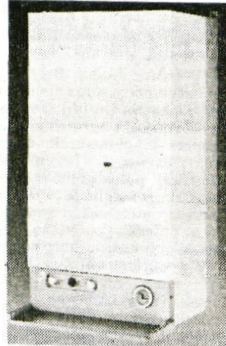
Iz programa Starclima je plinski stenski grelnik HYDRA 100/127 od 12.000 do 27.000 kcal/h. Ima bakreni izmenjevalec toplote za centralno ogrevanje in za pripravo tople vode. Izgorevalni prostor je iz keramičnih vlaken. Atmosferski grelec je izdelan iz nerjavečega jekla. Črpalka ima več hitrosti. Elektronska plošča usmerja, preverja in analizira signale. - HYDRA PLUS pa ima prostor za ventilacijsko skupino za prisilni vlek zunanjega zraka in odvod dimnih plinov.
