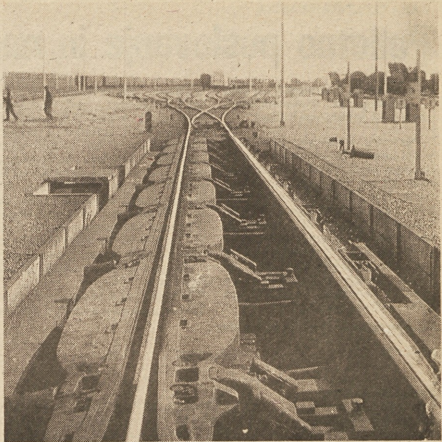
Našo serijo reportaž iz temeljnih organizacij združenega dela SOZD Iskra danes nadaljujemo z reportažo iz TOZD Inženiringi Industrije za avtomatiko v Ljubljani. Slika kaže zavoro za avtomatsko zaviranje na postaji Zalog pri Ljubljani.
