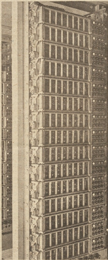
Stojalo z relejnimi skupinami signalne naprave.
