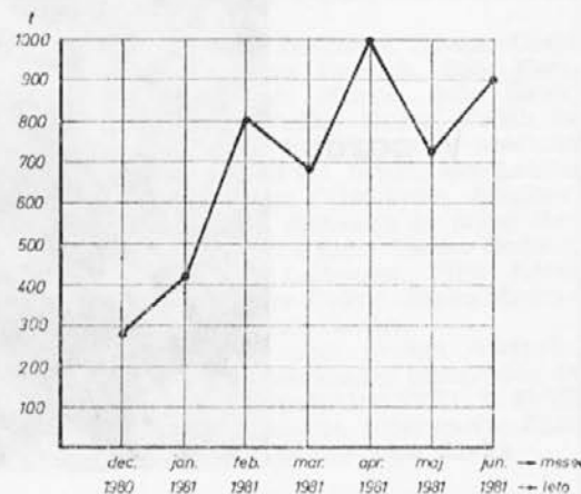
Slika 1: Proizvodnja kovaške linije SXP 40
