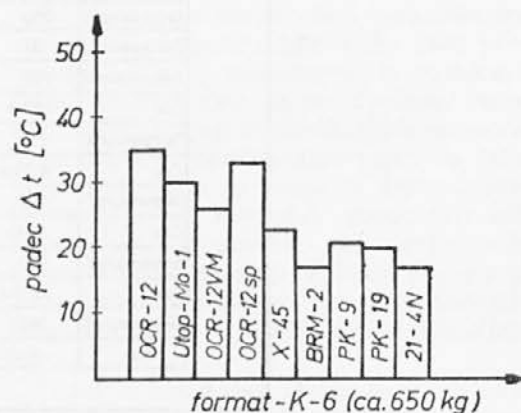
Slika 5: Padec temperature na poti od peči do kovaškega stroja za različne vrste jekel
