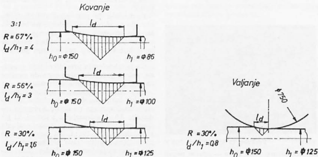
Slika 10: Primerjava preoblikovanja na kovaškem stroju in pri klasičnem valjanju
