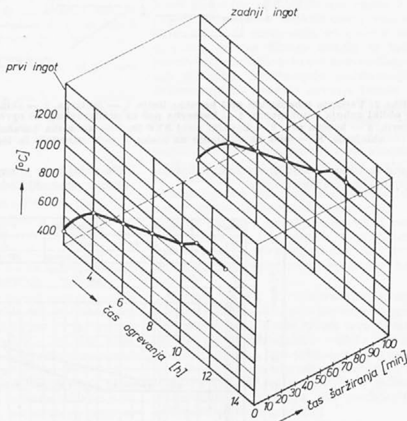
Slika 4: Diagram ogrevanja za prvi in zadnji ingot v krožni peči
