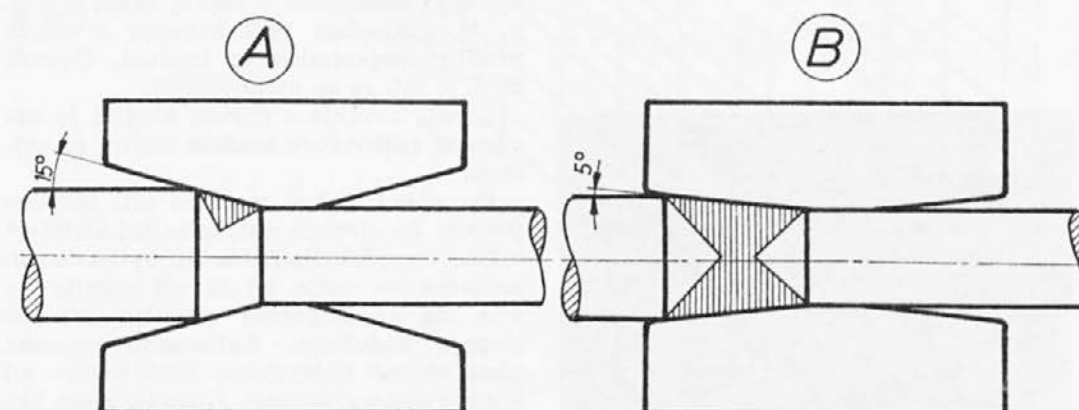
Slika 9: Shematičen prikaz vpliva geometrije kladiv na predelavo. A — Prevelik prijemni kot — premajhna redukcija — slaba predelava jedra, B — Pravilna izvedba prijemnega kota, ki omogoča globoko delovanje deformacij in zagotavlja dobro predelavo jedra
