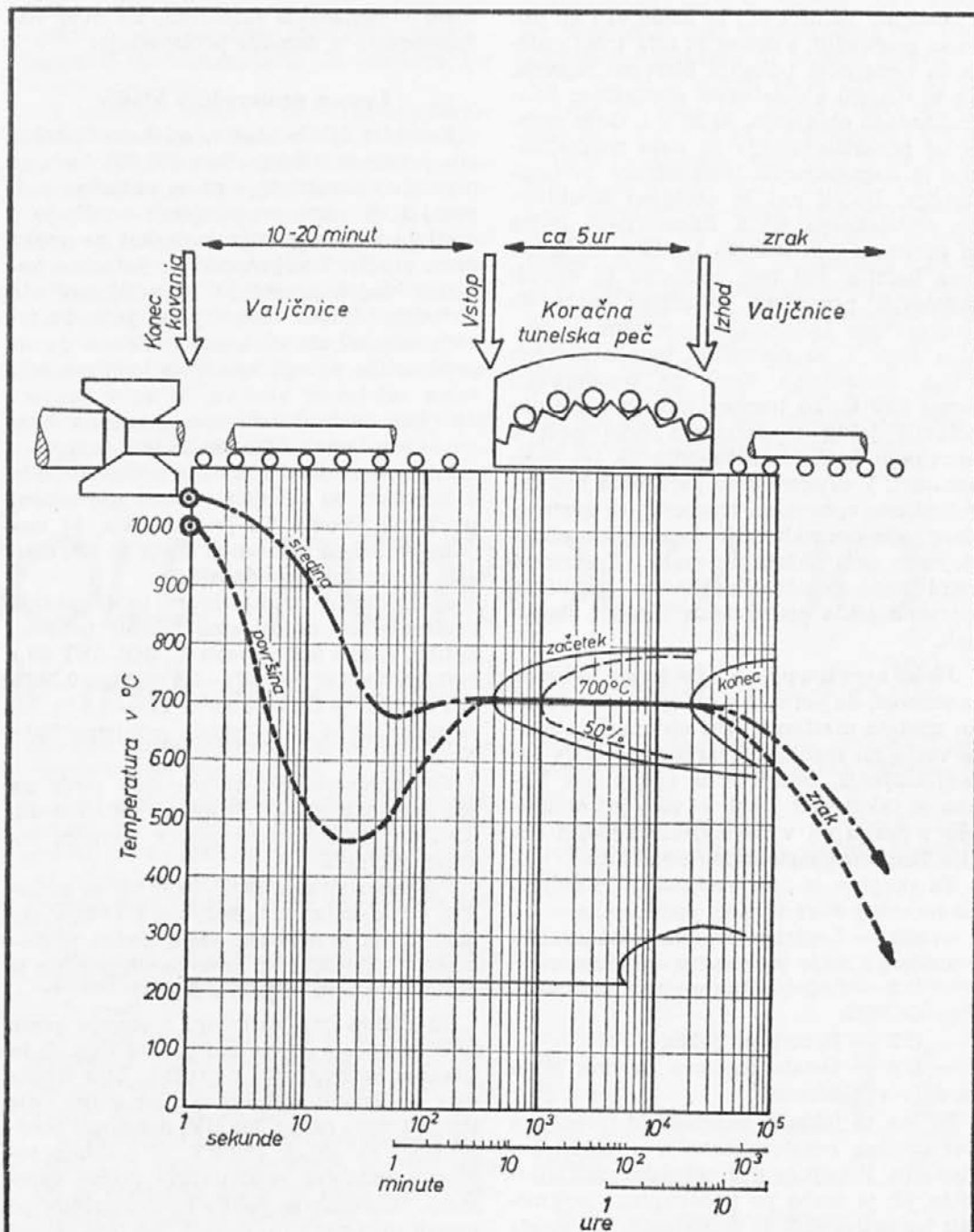
Slika 11: Princip kontroliranega ohlajanja z izotermalno premeno v perlitni stopnji
