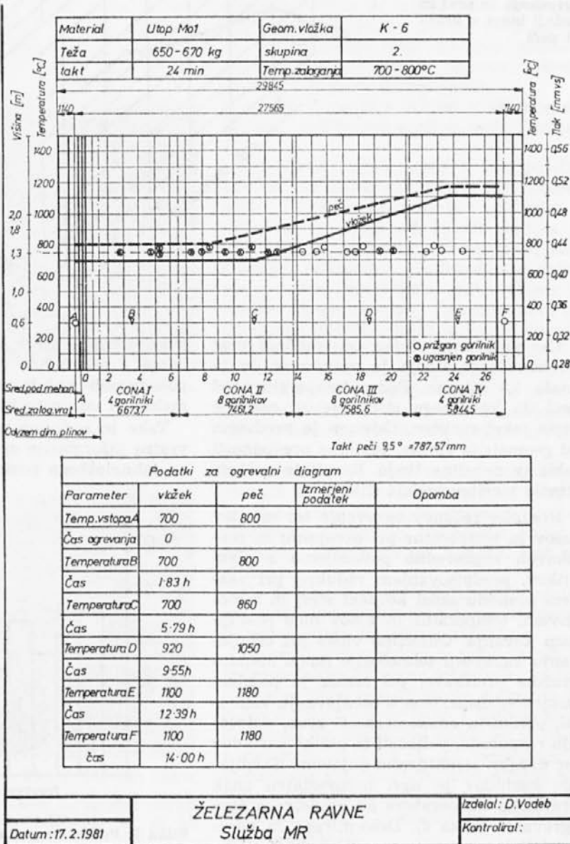
Slika 3: Primer predpisa ogrevanja v krožni peči kovaške linije
