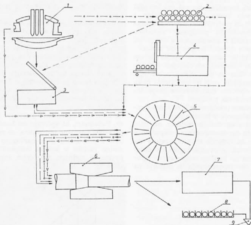
Slika 2: Variante tehnoloških poti kovaške linije. 1 — jeklarne, 2 — skladišče ingotov, 3 — peč v obliki zaboja s pokrovom, 4 — komorna peč za predgrevanje in ogrevanje v posebnih primerih, 5 — krožna peč, 6 — kovaški stroj SXP 40, 7 — tunelska koračna peč za kontrolirano ohlajanje, 8 — miza za ohlajanje na zraku, 9 — v adjustažo in toplotno obdelavo
