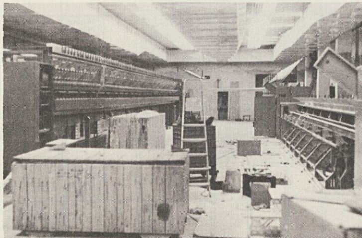
Levo avtomatski rotorski predilnik Ingolstadt za izdelavo OE preje. Desno, montaža dveh visokoproduktivnih flajerjev Zinser.
