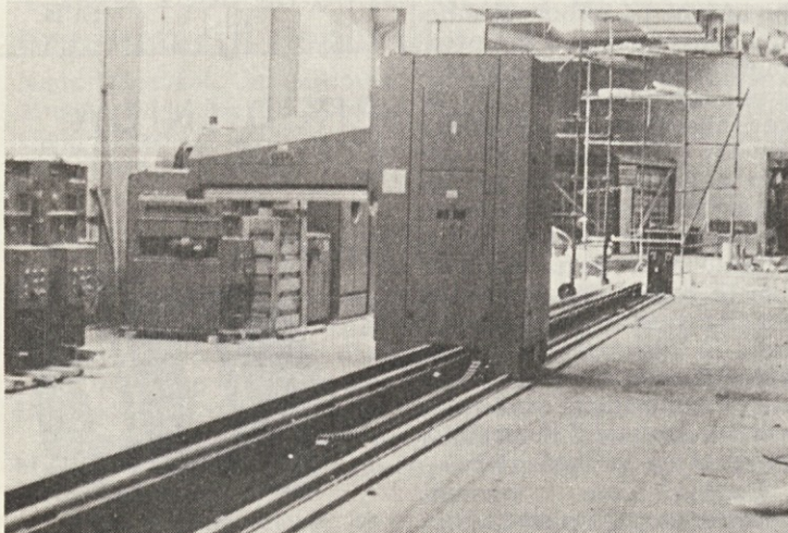
Montaža novega odzermalnika bal Hergeth (Optomix)
