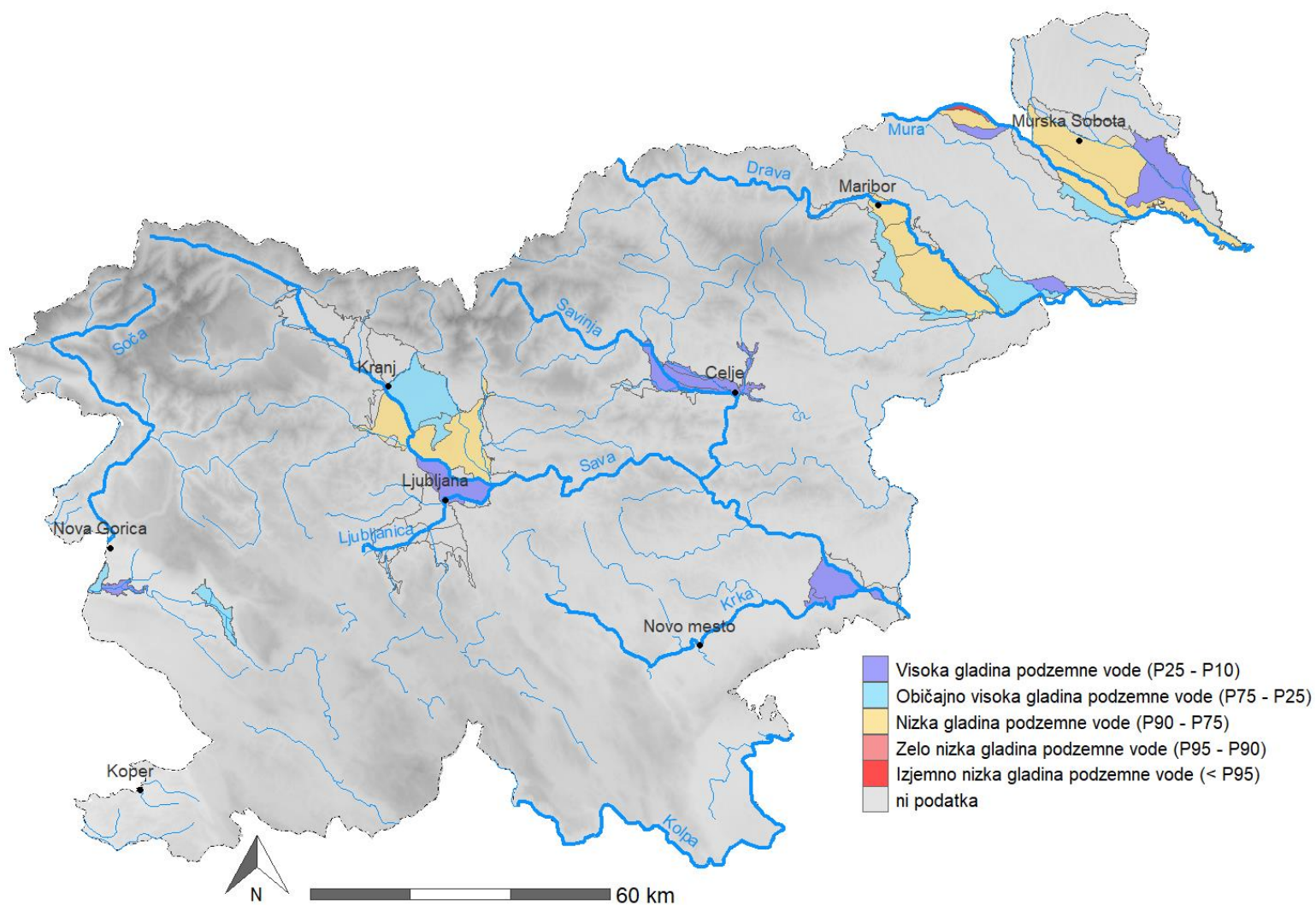
Slika 6. Uvrstitev povprečnih mesečnih gladin podzemne vode v medzrskih vodonosnikih v percentilne razrede gladin (P) referenčnega obdobja 1991–2020; december 2022 Figure 6. Average monthly groundwater level in alluvial aquifer classified in percentile values (P) of reference period 1991–2020; December 2022
