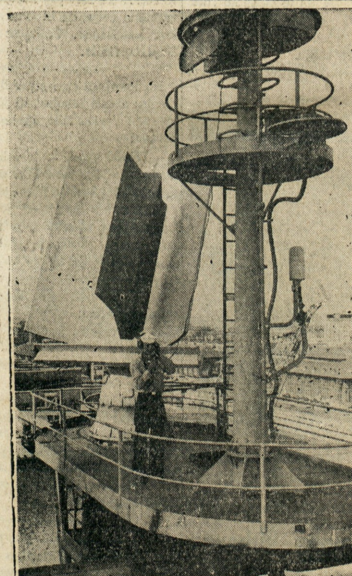
NOVOST — Hughes Aircraft Co. je izdelala novo vrsto lahke radarske antene, ki je elektronsko stabilizirana in je sposobna odkriti oddaljenost, velikost in višino naglo letječih letal. Na sliki jo vidimo na križarki Galveston v Fullertonu v Kaliforniji.
