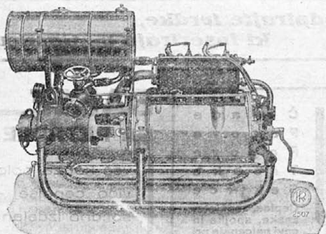
Dvocilindrska motorna brizgalnica, model 1929, 18/20 HP., pritisk do 16 atm. Hladilnik novega sistema, ogrevanje črpalke s toplo čisto vodo.
