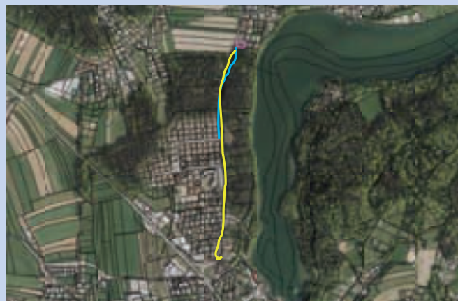
— trasa rekonstrukcije in gradnje kanalizacije za odpadno vodo — trasa gradnje vodovoda
