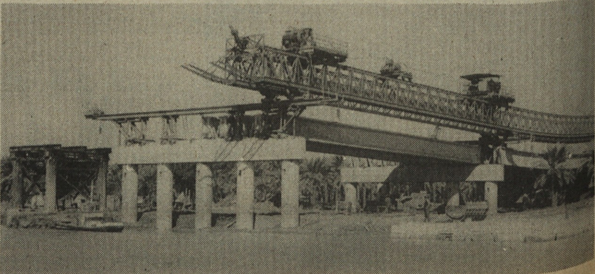
Montaža nosilcev v Amari
