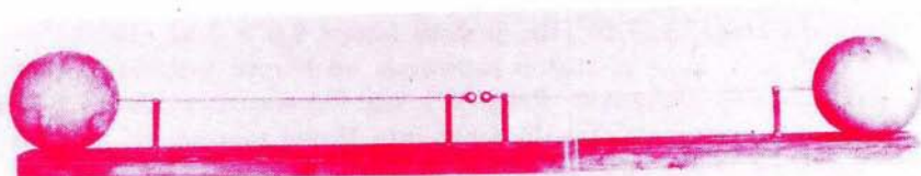
Slika 2. Risba oddajnega nihajnega kroga s tuljavo in oddajno anteno (zgoraj) in sprejemnega nihajnega kroga (spodaj) iz članka H. Hertzja O vplivu premočrtnega električnega nihanja na bližnji ovoj iz novembra 1887. Del Hertzove naprave so razstavili leta 1988 na univerzi v Karlsruheju na razstavi Sto let radijskih valov .
