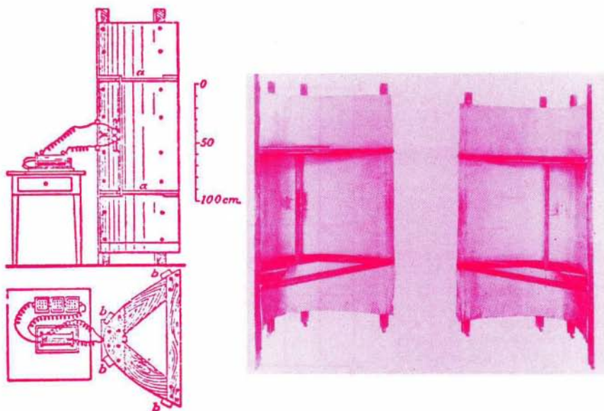
Slika 4. Risba izpopolnjenega oddajnega kroga z navpično anteno v gorišču parabolčnega zrcala (s strani in od zgoraj) iz Hertzevega članka O curkih električne sile iz leta 1889 in pločevinasti zrcali oddajne in sprejemne antene.
