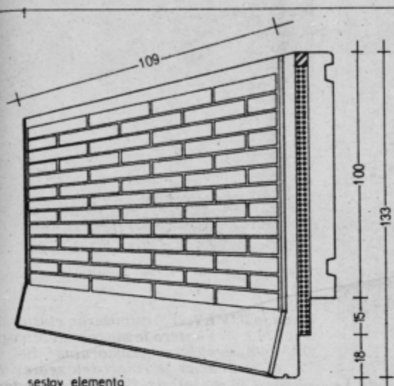
sestav elementa
