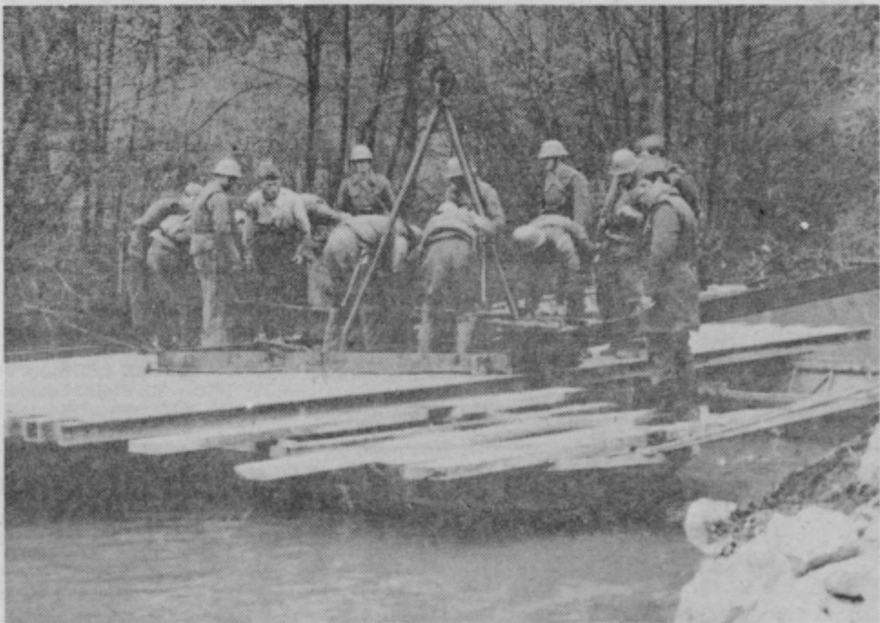
Zaradi muljastega dna so morali inženirci iz enote Mileta Krstića zabiti pilote 3 metre v dno. Kljub pomanjkanju materiala vojaki delajo zavzeto.
