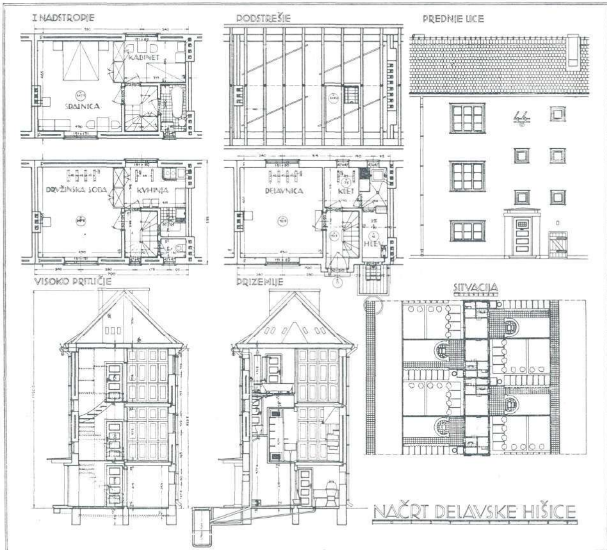
Iv. Vurnik: Načrt delavske hiše 2/I
