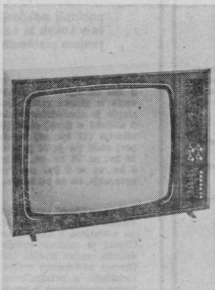
Črno-beli televizor Iskra PANORAMA ARIES: tiskano vezje, 10 elektronk, 7 tranzistorjev, 21 diod, VHF in UHF kanalnik, ekran 61 cm
