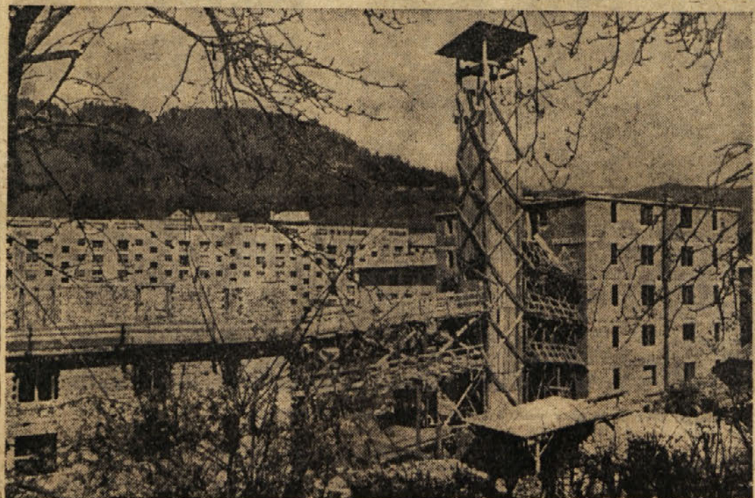
Gradnja stanovanjskih stolpičev v Trbovljah, ki jih gradi Splošno gradbeno podjetje »Zasavje« — Trbovlje — v osrednju K-4
