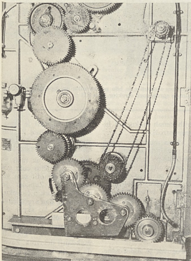
Flyerska krila sedaj poganjajo zobčniki, ki so jih konstruirali in izdelali naši delavci
