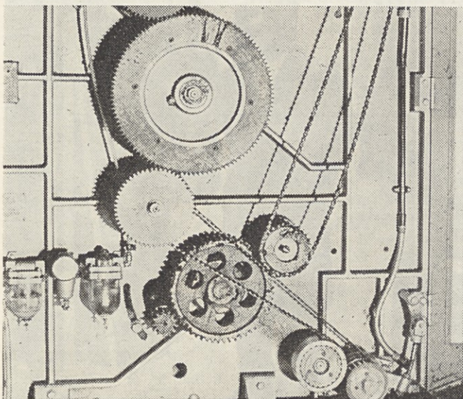
Tu vidimo pogon z jermenom, kjer je prihajalo do pogostih zastojev zaradi številnih menjav ležajev
