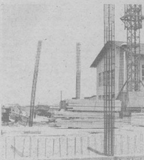
Pri osnovni šoli Stane Kosec v KS Edvard Kardelj gradijo prizidek s 4 učilnicami, telovadnico in večnamenskim prostorom. Za celodnevno osnovno šolo, ki jo obiskuje več kot 400 učencev, bo to vsekakor velika pridobitev.
