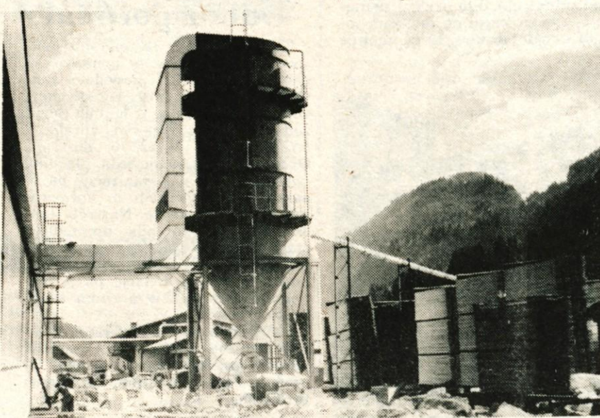
V tovarni za masivno predelavo lesa v Alpesu Železniki so tako kot v drugih Alpsovih tovarnah poskrbeli za čist zrak v proizvodnih halah. Posebna odsesovalna naprava sesa zrak iz delavnice skupaj z lesnimi drobtinami, ga v posebnem valju filtrira in ga vrača v proizvodno halo. S tem dosežejo na eni strani boljše delovne pogoje in prihranijo pri ogrevanju, ker topel zrak stalno kroži. (lb) - Foto: F. Perdan
