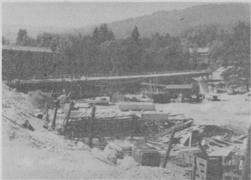
Po Hünnebeck sistemu, oziroma po sistemu premičnih opažev raste nov most v Radečah.
