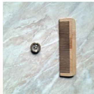
knof, kampl
