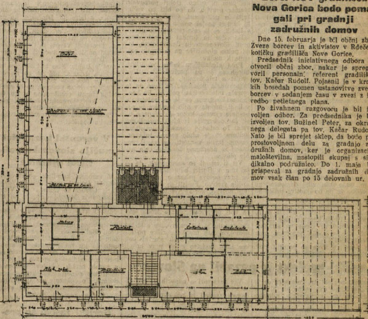
Tloris I. nadstropja zadružnega doma v Oseku
