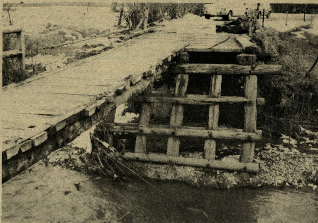
Te dni so pričeli obnavljati most čez Bolsko v Čepļah. Stari leseni most je delno odnesla zadnja jesenska poplava. Krajanji so ga usposobili le za pešce, ne pa tudi za vozila. Most bodo obnovili z občinskimi sredstvi. Gradbena dela bodo stala 600 tisoč dinarjev. Na sliki: Tako je izgledal del starega mostu pred dnevi.
