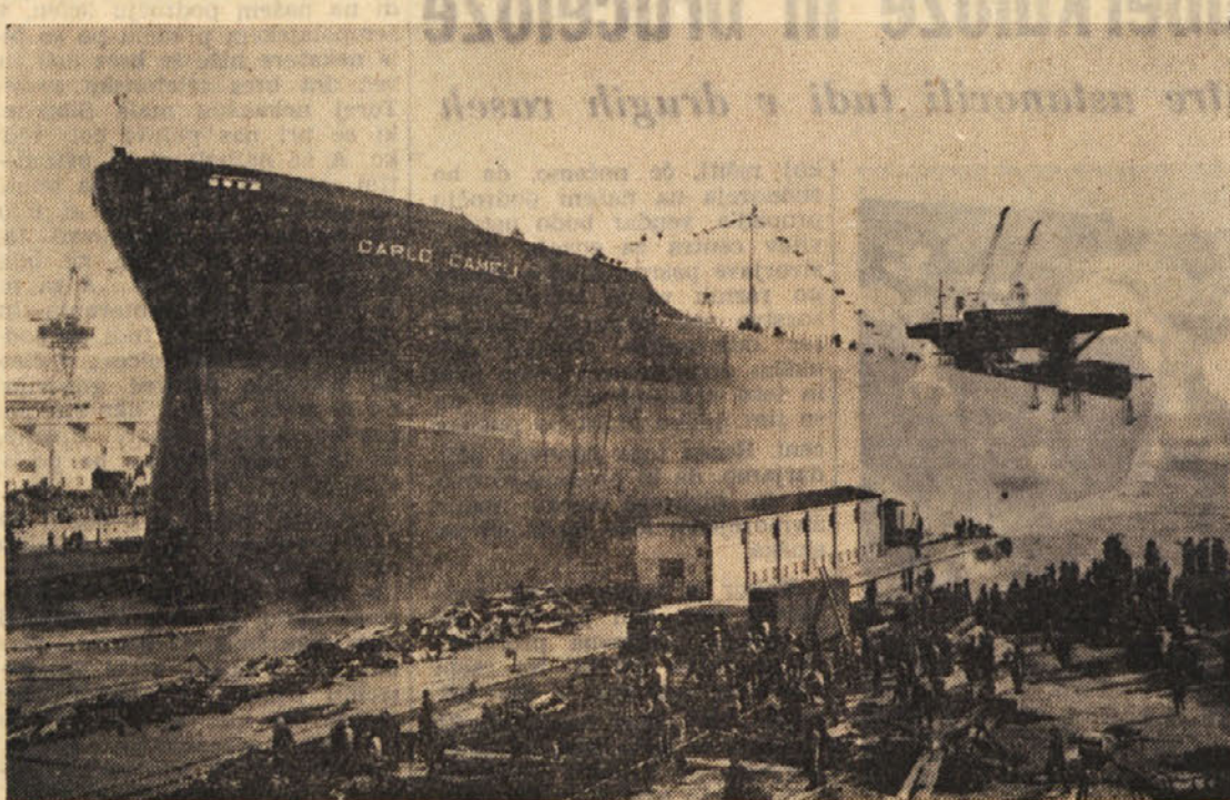
Ogromen trup motocisterne "Carlo Camelli" zanesljivo drsi v objem morja
