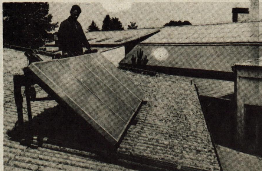
Stirje sončni kolektorji na strehi Zavoda za hlajenje in klimatizacijo na Trati pri Škofji Loki bodo omogočili številne praktične raziskave o tem, kako je v naših vremenskih razmerah mogoče uporabljati sončno energijo za ogrevanje vode. — Foto: F. Perdan
