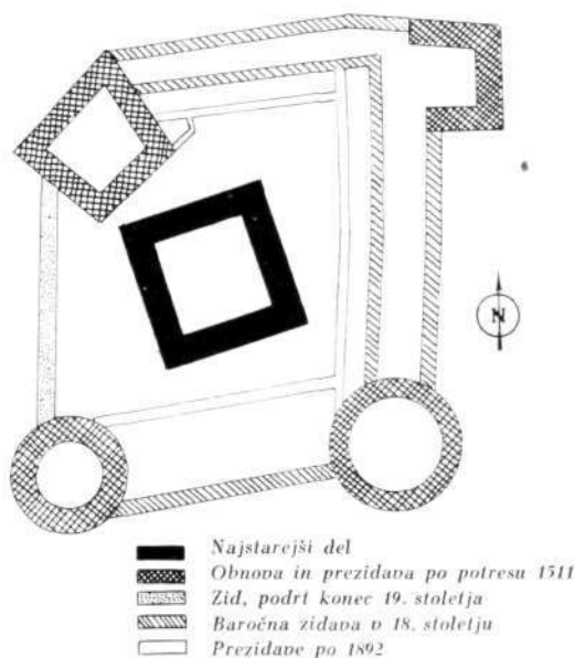
Shematični tloris loškega gradu (narisal F. Stukl)
