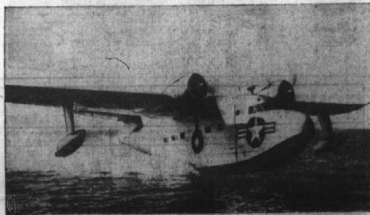
Slika nam kaže najnovejšo mornariško letalo, ki se lahko dvigne z vodne gladine ali s suhe zemlje v zrak. To je Grumman Albatross, ki ima tri moze posadke in lahko nese 14 potnikov ali 4.100 funtov tovora. Čez Atlantski ocean leti s hitrostjo 225 milj na uro brez pristanka od 600 do 1.400 milj.
