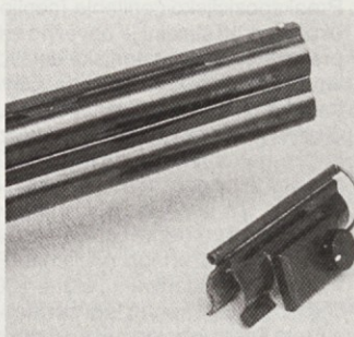
Svetlobni vizirček, ki tehta le 45 g, je mogoče z vodili v obliki objemke enostavno pritrditi na cev šibrenice.
