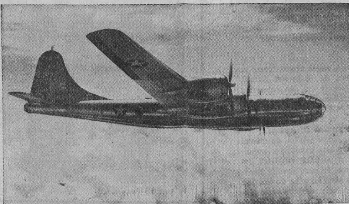
Slika nam predstavlja veliko zračno trdnjavo tipa Boeing B-29, s kakršnimi naši fantje napadajo Japonce. Preko kril meri 141,2 čevljev, je 98 čevljev dolga in 27 čevljev visoka; ima štiri Wright Cyclon motorje z 2000 konjskimi silami, leti z bržino 300 milj na uro in v višini 30.000 čevljev.
