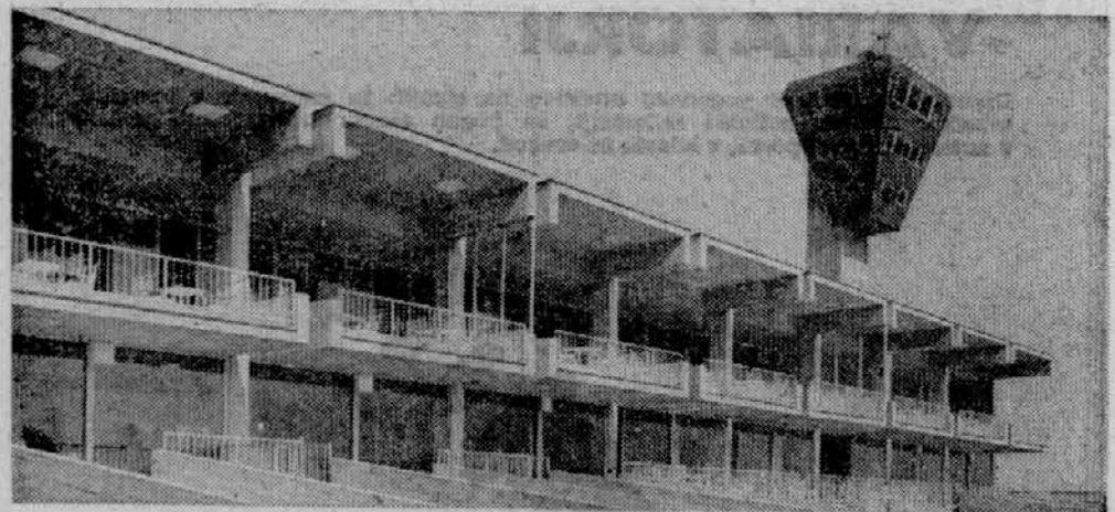
Pristaniška zgradba letališča Omišalj na otoku Krku
