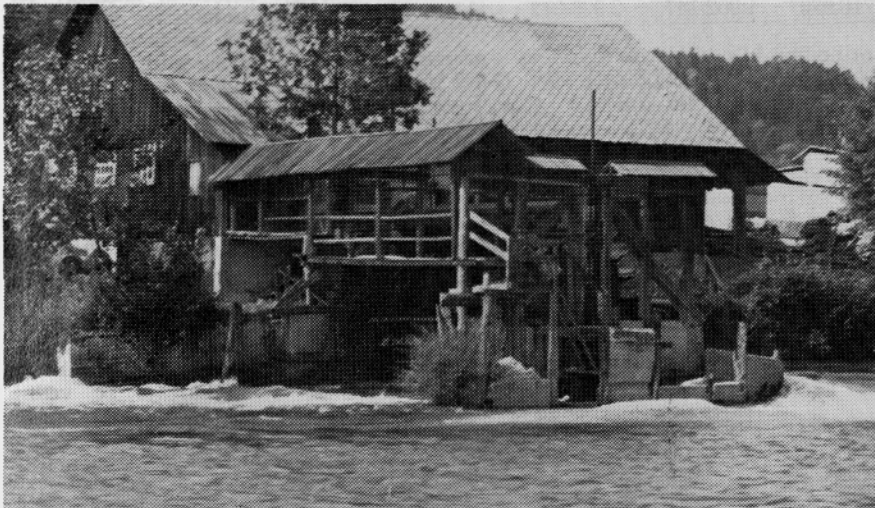
Stara žaga v Podnartu s polnojarmenikom, ki je obratovala do leta 1965
