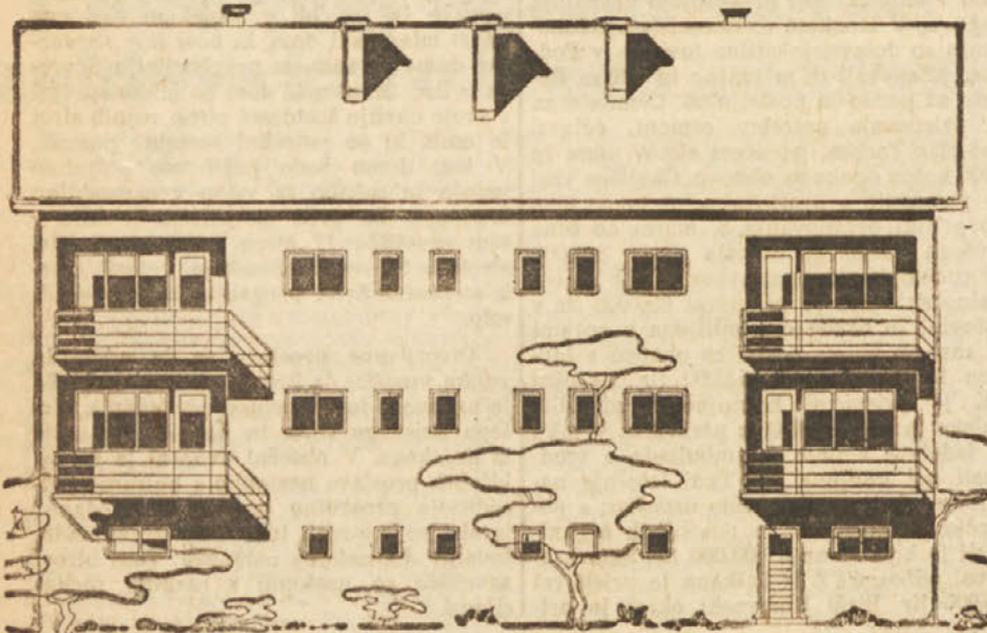
ZAHODNA FASADA
