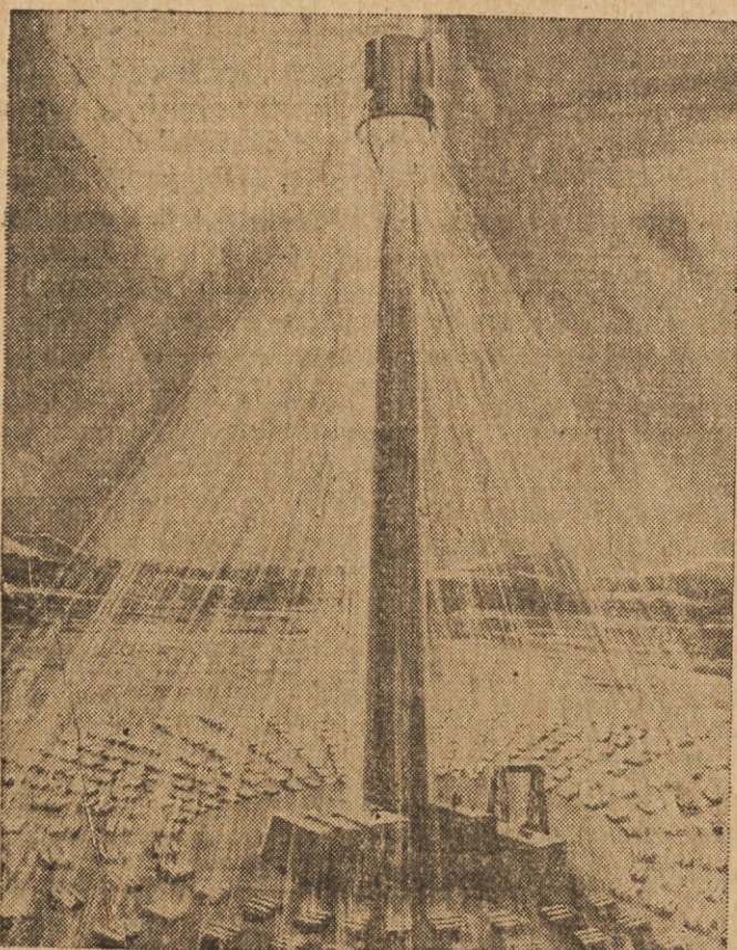
"STOLP ENERGIJE" — Honeywell raziskuje po naročilu Administracije za preiskave in razvoj energetskih virov "stolp energije", ki ga kaže gornja slika. Na vrhu stolpa je kotel z vodo, na katerega je usmerjena vrsta zrcal, ki s pomočjo sončnih žarkov segrevajo vodo in jo spremenjajo v paro. Paro uporabljajo pod stolpom za pogon turbinskega generatorja.
