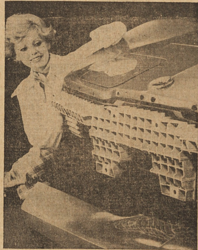
PROŽNA MREŽA — Na sliki je prednji del avtomobila, ki ima spredaj varnostno mrežo s prožno oporo. Če se avto zadene, se odbijača vda, pa se nato zopet vrne na svoje mesto brez vsake škode.
