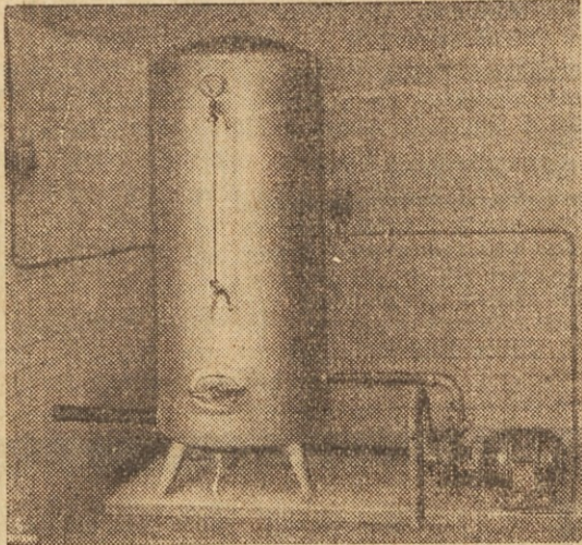
Selbsttätige Wasserringpumpe mit Druckkessel von 300 Liter Inhalt
