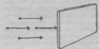
Beta delci
