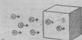
Nevtroni
