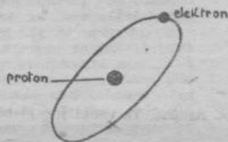
Vodikov atom
