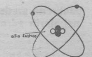
Helijev atom
