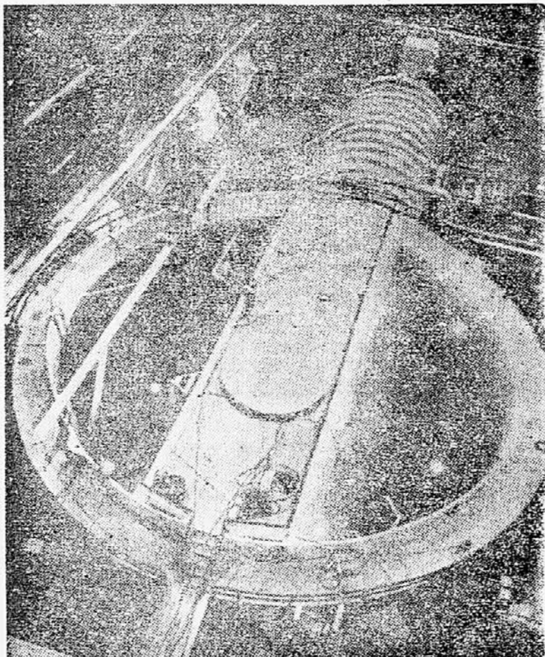
Slika prikazuje montažo atomskega reaktorja v tanker. Reaktor zavzame zelo veliko prostora zaradi zaščitnega oklepa, ki mora zadrževati nevarne žarke. Prostor so pridobili s tem, ker na taki ladji ni skladišča za premog ali nafto. Konstruktorji pa še niso povedali, kaj bi se zgodilo z radioaktivnim reaktorjem v primeru brodoloma...
