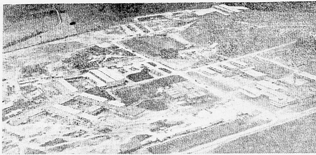
Gradnja laboratorijev Evropske organizacije za raziskovanja nuklearne energije v Meyrunu pri Zenevi je zelo napredovala. Slika kaže desno zgoraj z zemljo zasuti kanal 25-GeV-Protosinhrotrona. Nad njim je velika dvorana za poskuse. V sredini je sinhrociklotronska dvorana za 600 milijonov elektrovoltoev, ki že obratuje. Konstrukcija te dvorane je arhitektonska posebnost. Levo so osrednje delavnice in upravna poslopja. Na skrajni desni je električna centrala s kurilnico.
