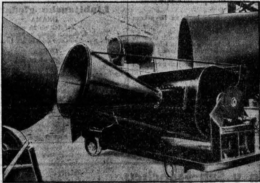
L'apparecchio Röntgen per l'esame dell'acciaio. — Röntgenski aparat za preiskovanje jekla.
